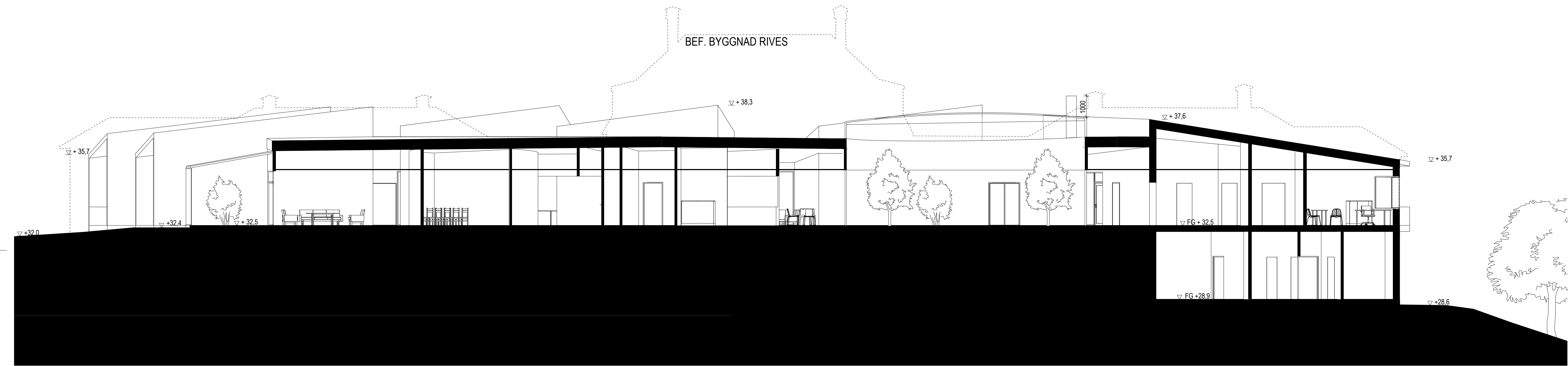
LÄNGDSEKTION C-C
